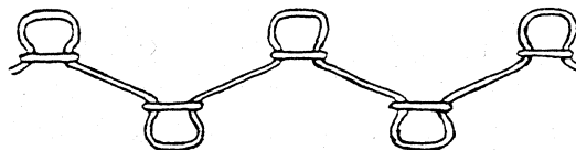
Рис. 5 Трикотажное полотно переплетения ластик типа 1 лицевая петля x 1 петля, снятая без провязывания
