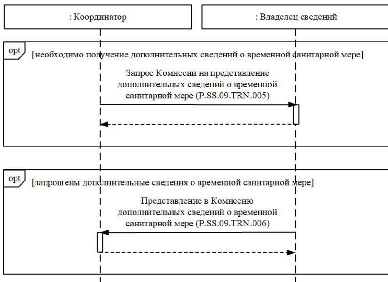
Рис. 4. Схема выполнения транзакций общего процесса при получении Комиссией дополнительных сведений о временной санитарной мере
