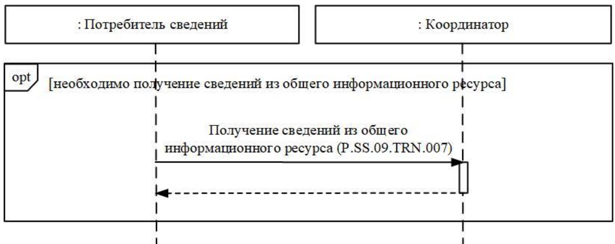
Рис. 5. Схема выполнения транзакций общего процесса при получении сведений из общего информационного ресурса
