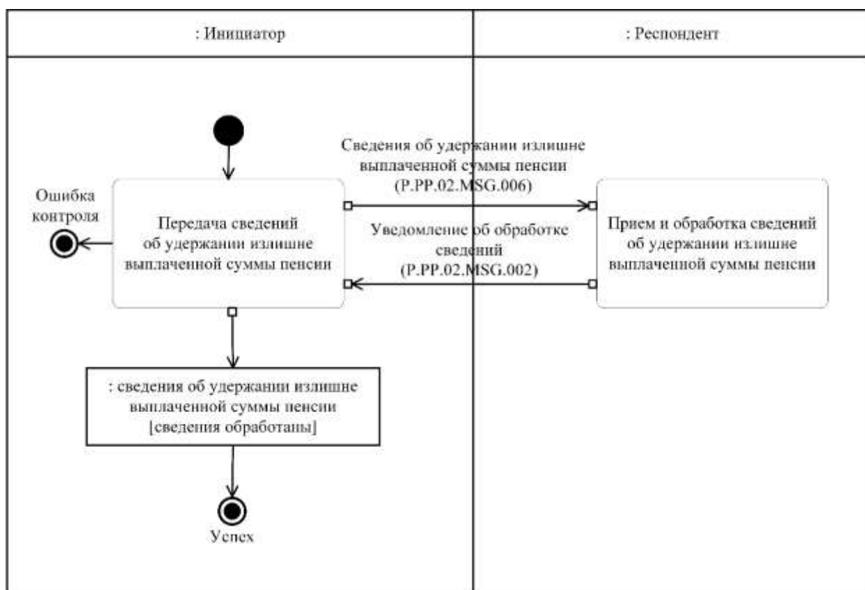
Рис. 8. Схема выполнения транзакции общего процесса «Представление сведений об удержании излишне выплаченной суммы пенсии» (P.PP.02.TRN.005)
